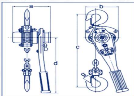
Palancas Serie VR2 Marca Vital
